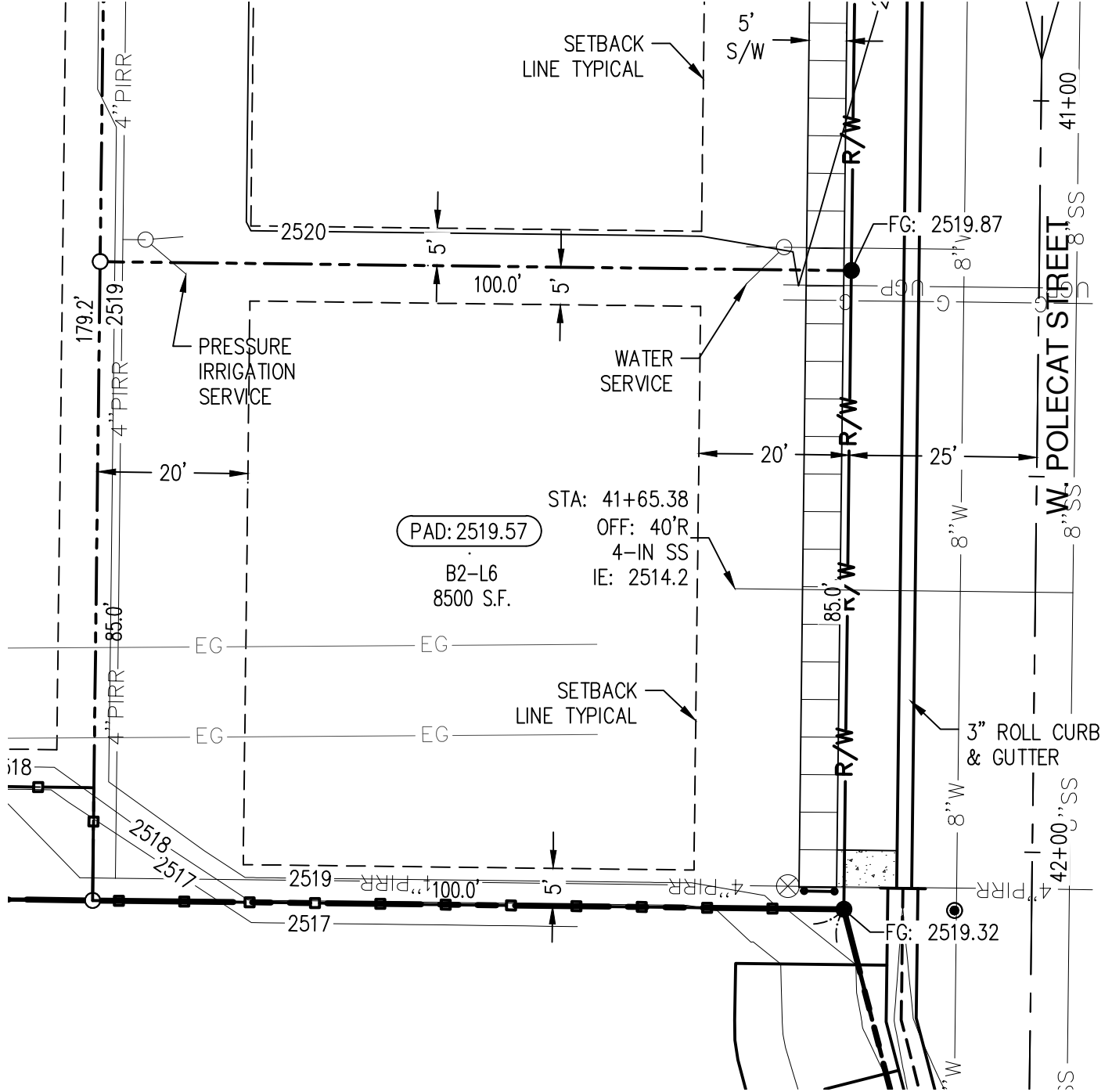
PLAN HORIZONTAL SCALE: 1" = 20'
